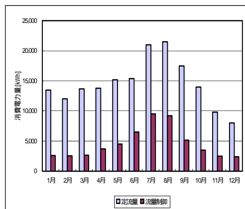
図6 定流量(導入前)と流量制御時(導入後)の月別消費電力量
