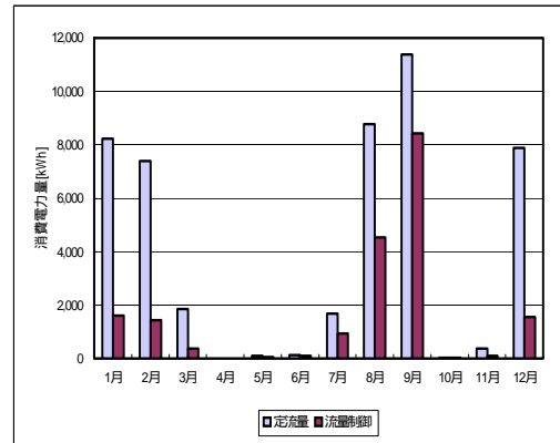
図4 定流量(導入前)と流量制御時(導入後)の月別消費電力量
