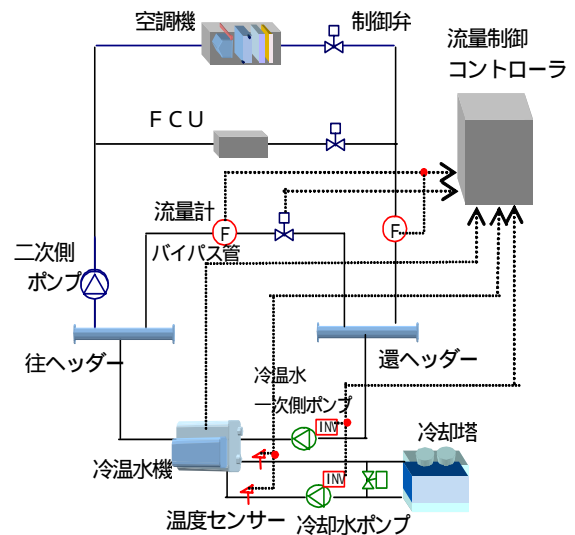
図2 流量制御システム導入後のフロー図
