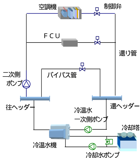
図1 従来方式のフロー図
